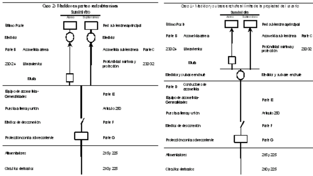
Figura 230-1.- Acometidas
