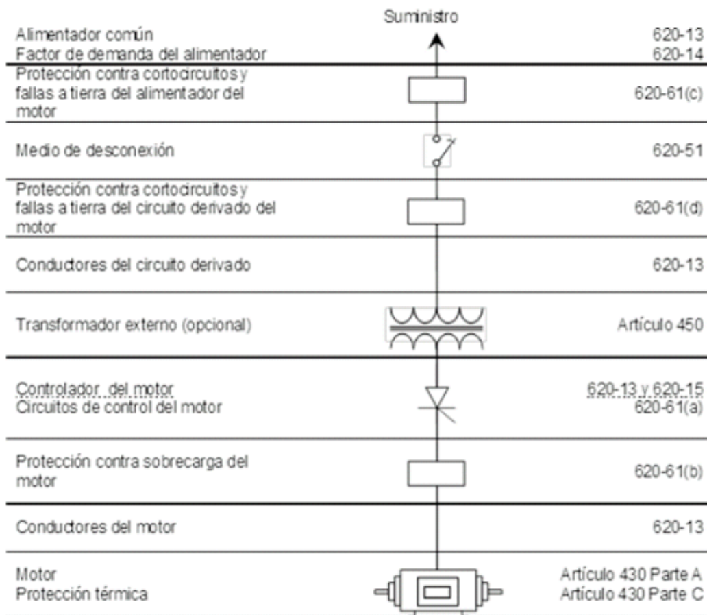
Figura 620-13.- Diagrama unifilar
